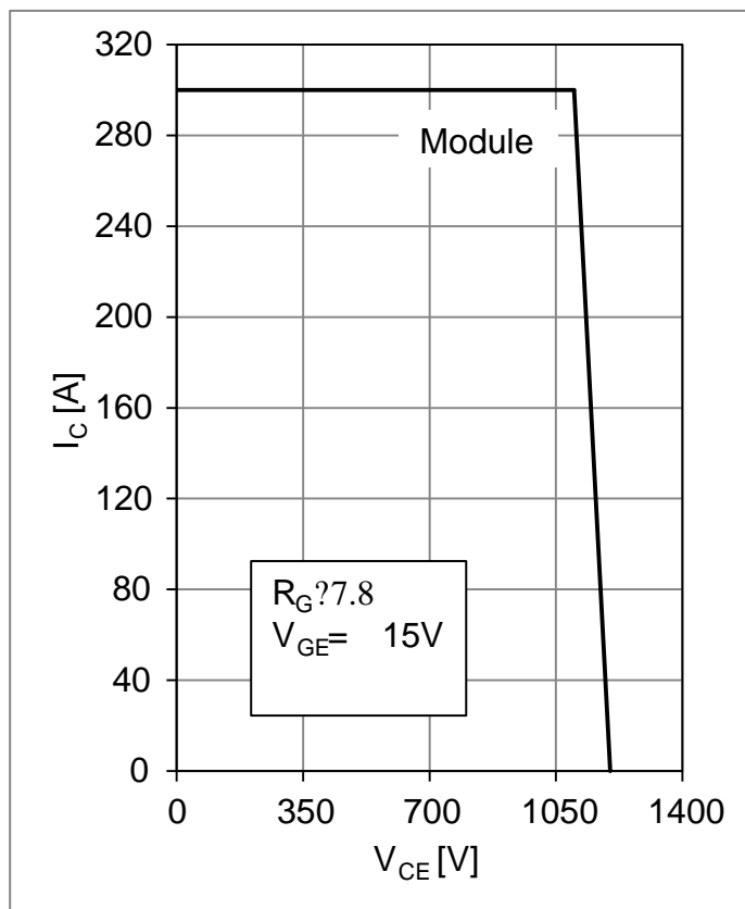
Fig 5.RBSOA
